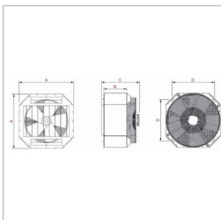
Schéma Destratificateur Spot
